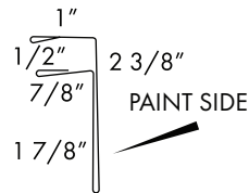
F-TRIM
