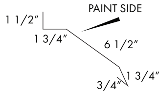
FASCIA TRIM
