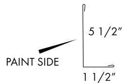
F-TRIM
