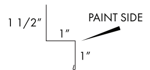
C-TRIM
